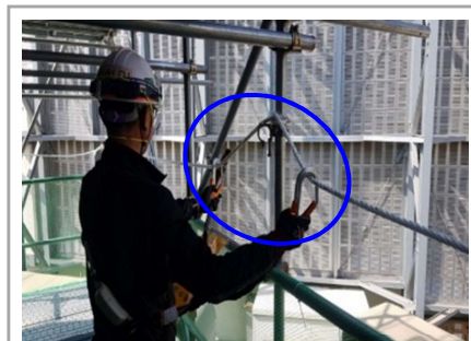
안전대 걸이시설 / 더블 Hook(권고)
