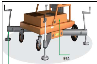
아웃트리거
