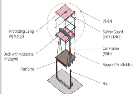
임시카 구조
